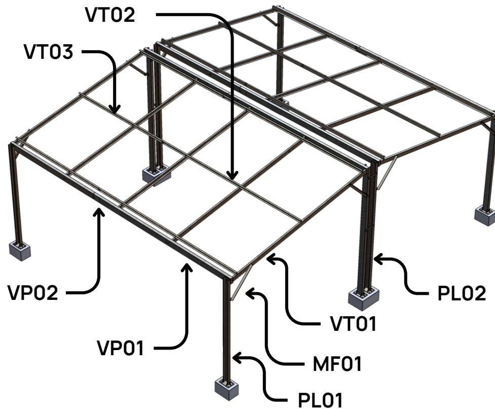
VISTA ISOMETRICA
